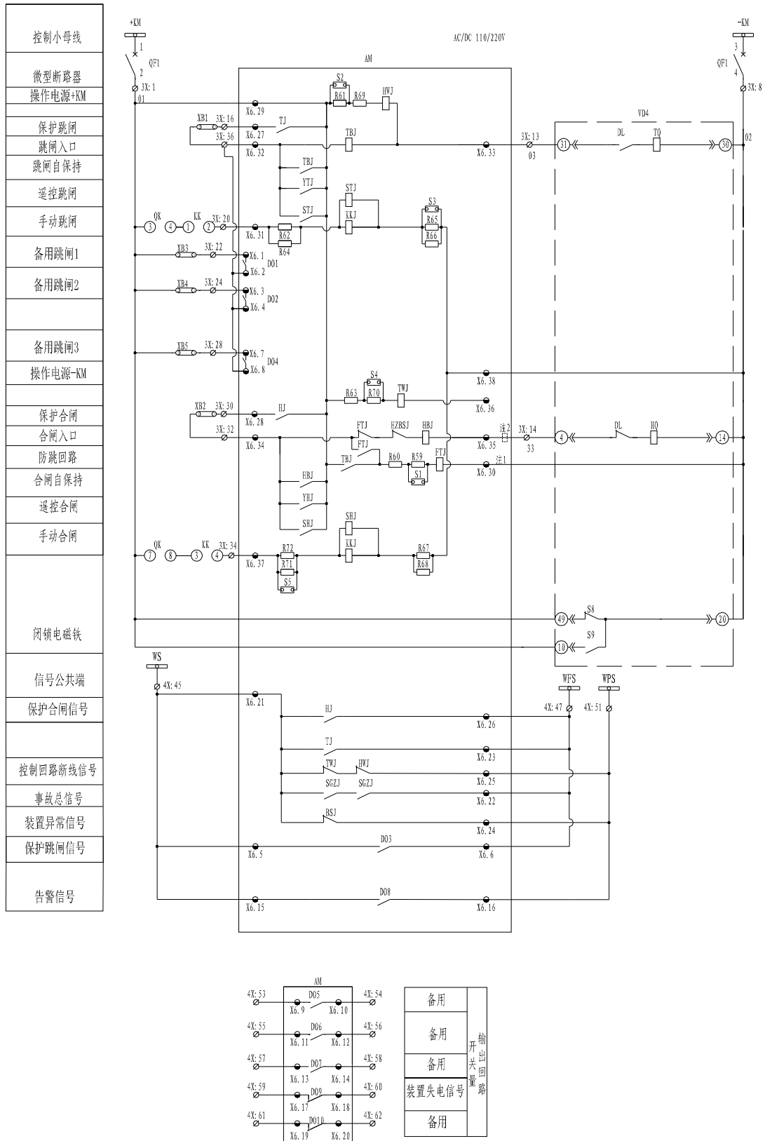
图 1.26 AM5-M-Q 二次原理图 (三)
