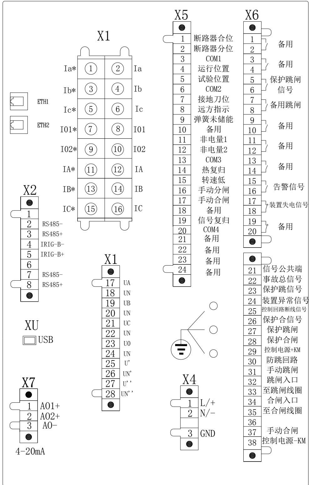
图 1.22 AM5-M-Q 电气接线图
