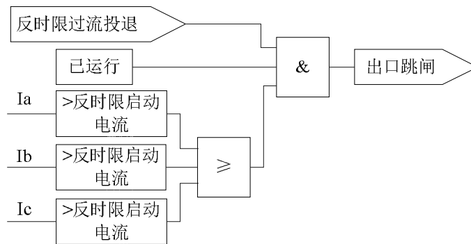
图 1.3 反时限过流保护逻辑
