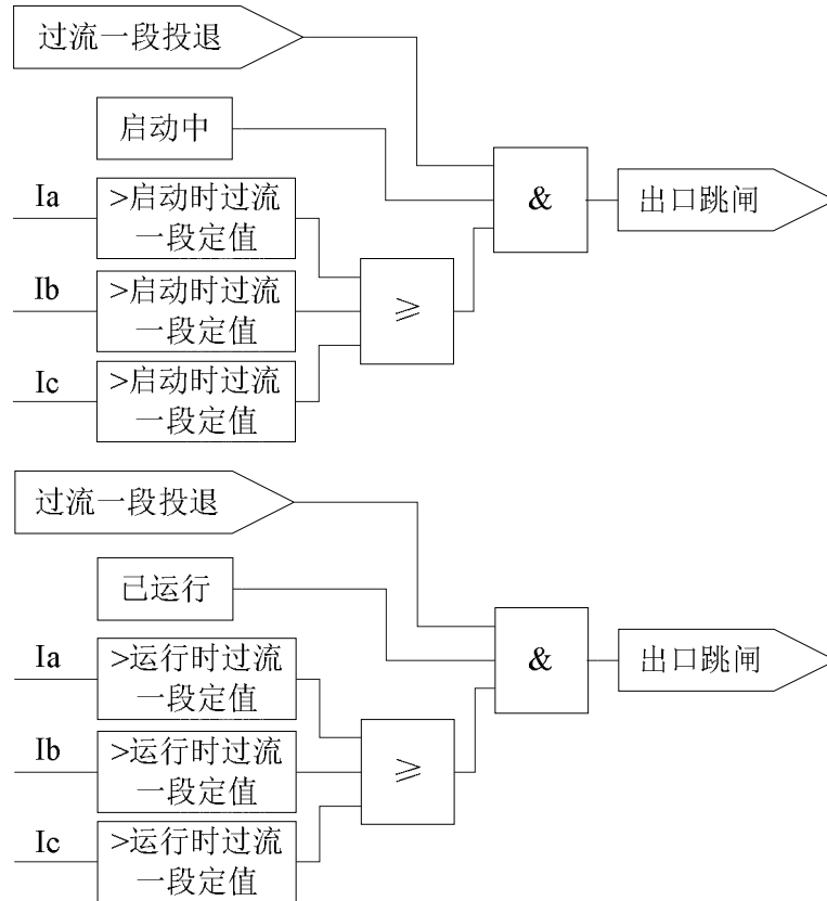
图 1.1 过流一段保护逻辑
