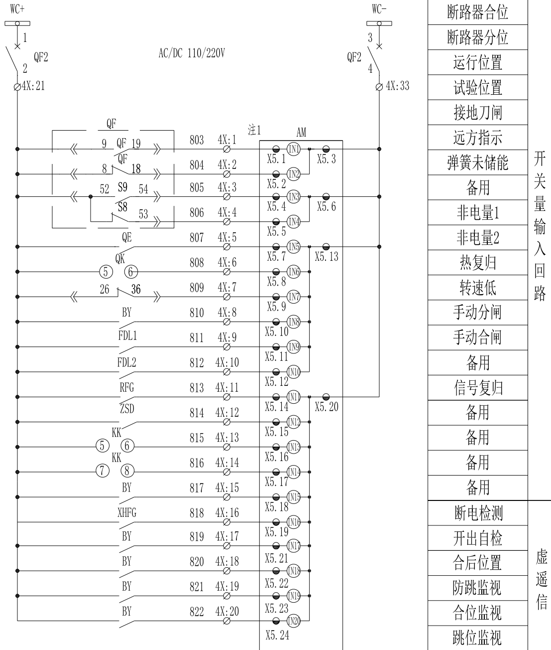
图 1.25 AM5-M-Q 二次原理图 (二)
