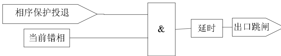
图 1.19 相序保护逻辑
