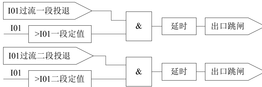
图 1.6 两段式零序过流保护逻辑
