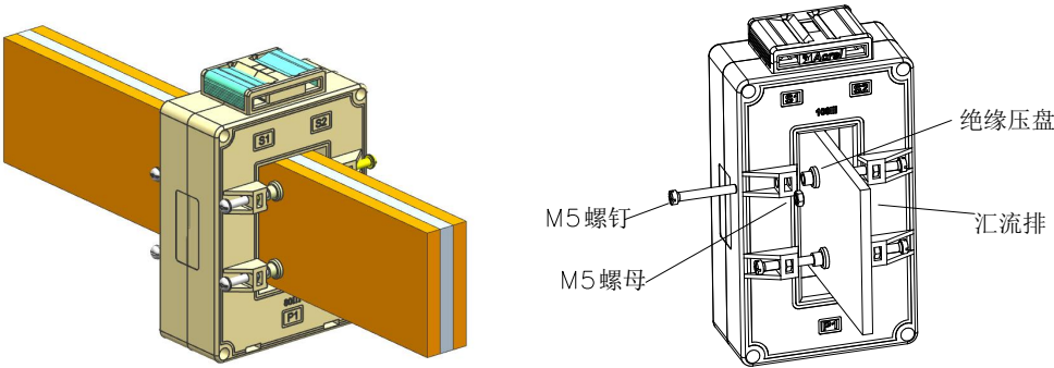
E. 母线固定
