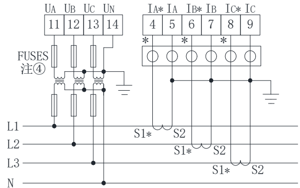
3P4L/3PT+3CT (仪表设置为3P4L)
