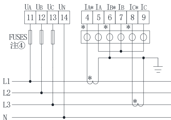
3P4W/2CT (仪表设置为3P4W) 注②
