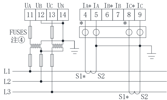
3P3L/2PT+2CT-1 (仪表设置为3P3L)
