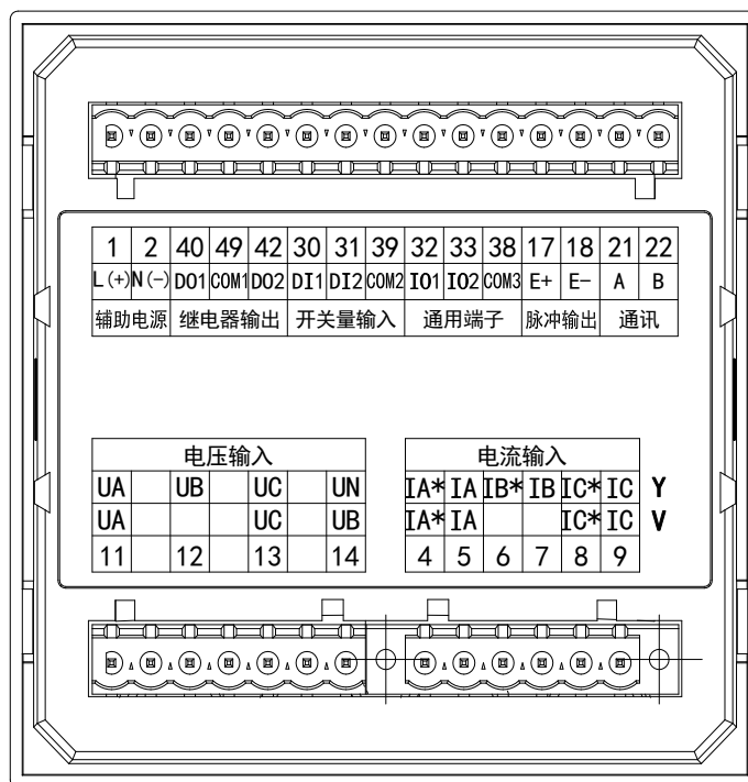
图 8 AMC96 系列接线端子图
