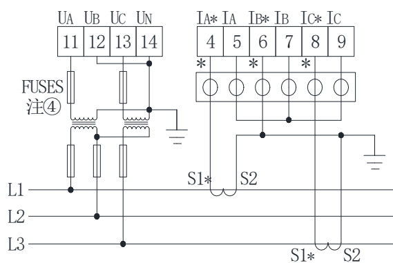
3P3L/2PT+2CT-2 (仪表设置为3P3L) 注③
