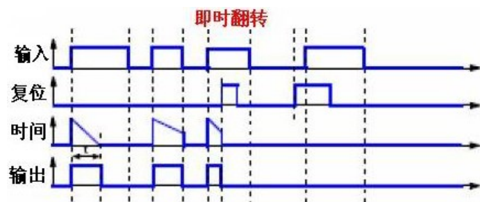
图 29 即时翻转定时器动作图
